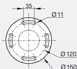
Typ/mod. BOS3-CDH-1AFO
