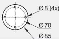
Typ/mod. BOS3-CDH-1ZFE
